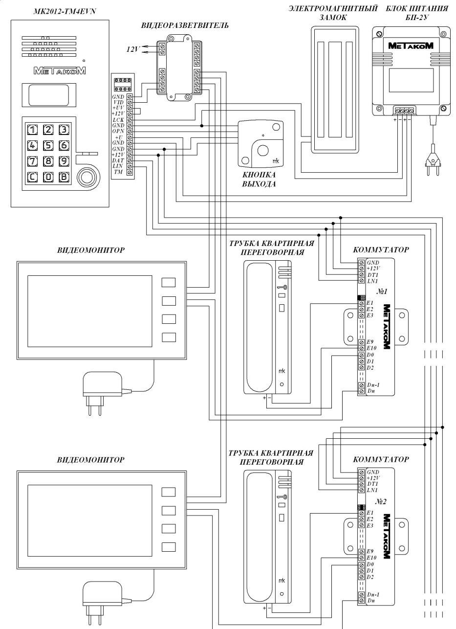
Рис. 2 Пример монтажа блока вызова МК2012-ТМ4ЕVN
