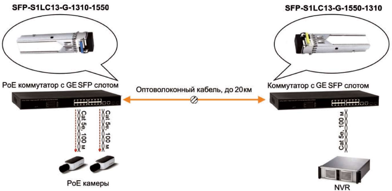
Рис.8 Типовая схема подключения SFP модулей SFP-S1LC13-G-1310-1550, SFP-S1LC13-G-1550-1310
