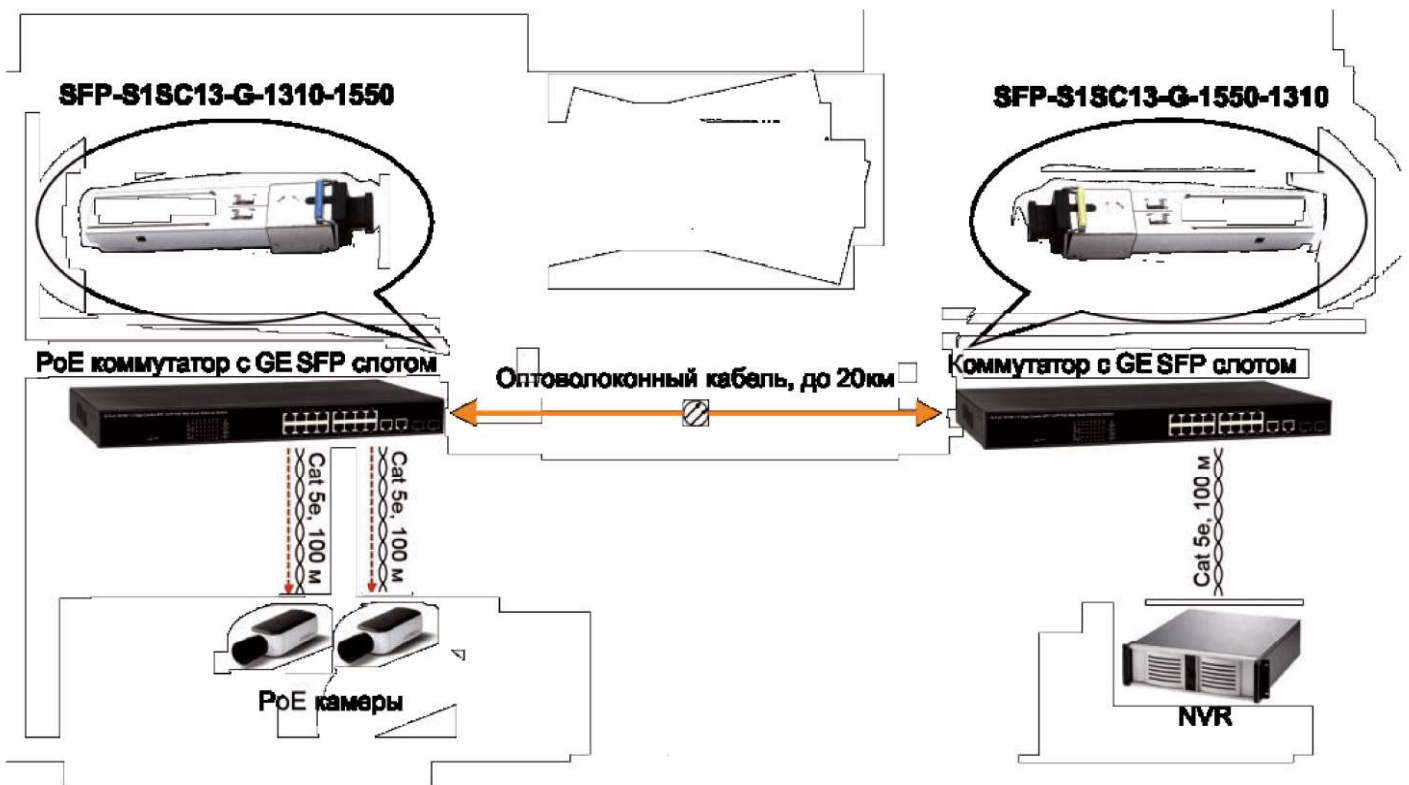
Рис.6 Типовая схема подключения SFP модулей SFP-S1SC13-G-1310-1550, SFP-S1SC13-G-1550-1310
