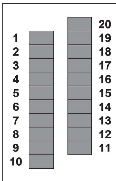
Рис. 5 Распиновка SFP разъема
