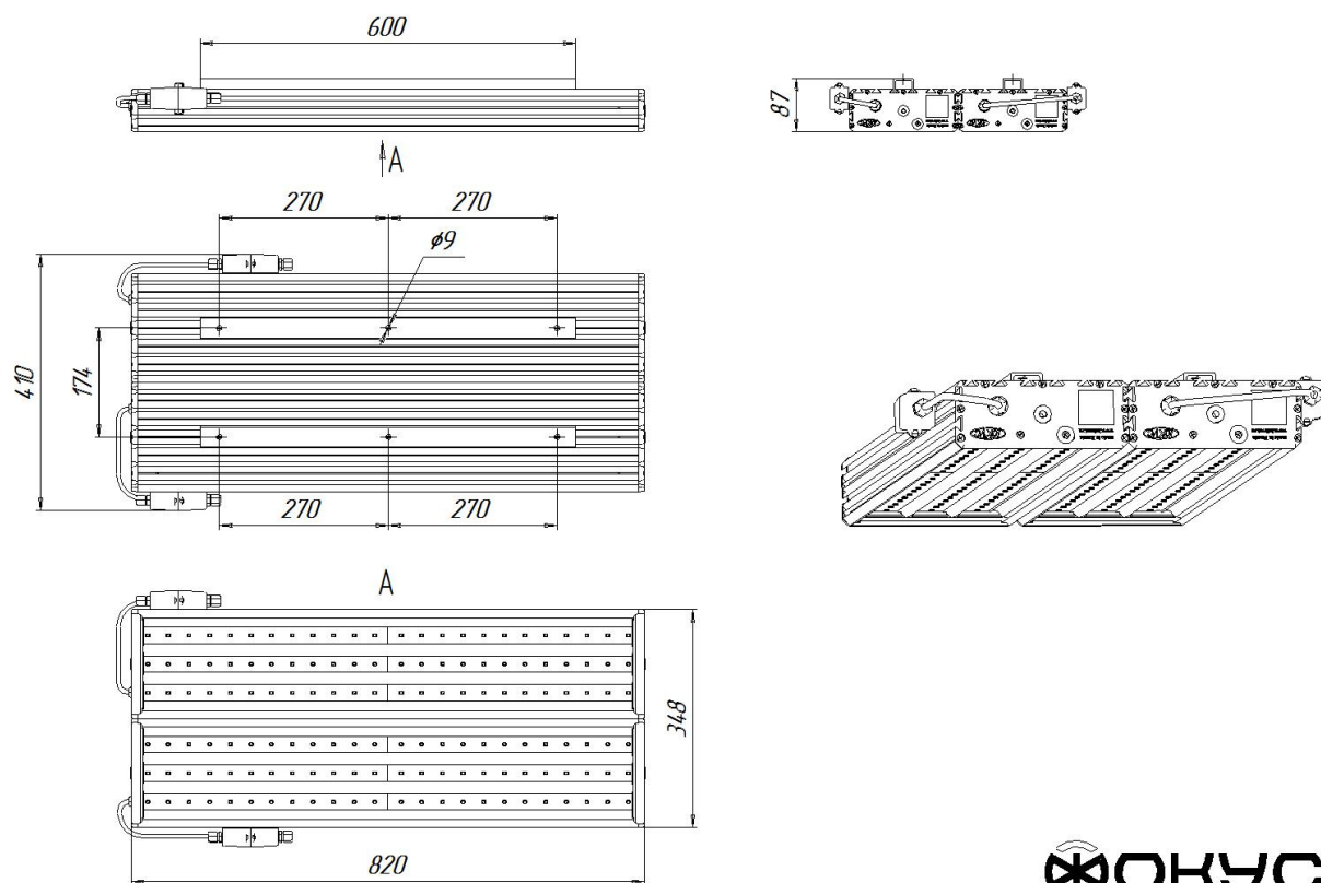
Светильник УСС 150 потолочное крепление
