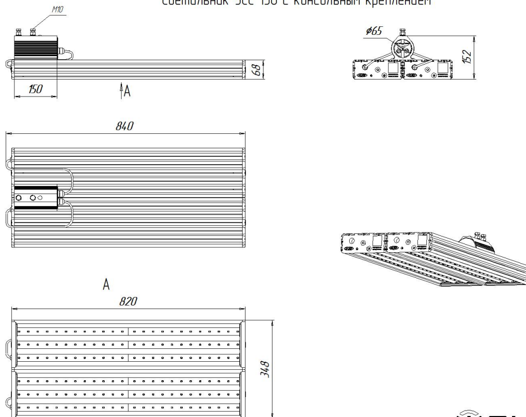
Светильник УСС 150 с консольным креплением
