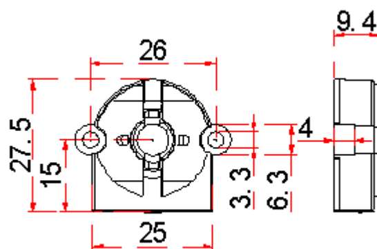
Патрон (ламподержатель) G13 торцевой, встраиваемый, w 9,4mm, для люминесцентной лампы T8, крепление на винт (акс.угловой кронштейн 15.013)
