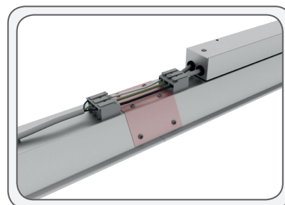
Просто соединять, светильники соединяются при помощи торцевого переходника.
