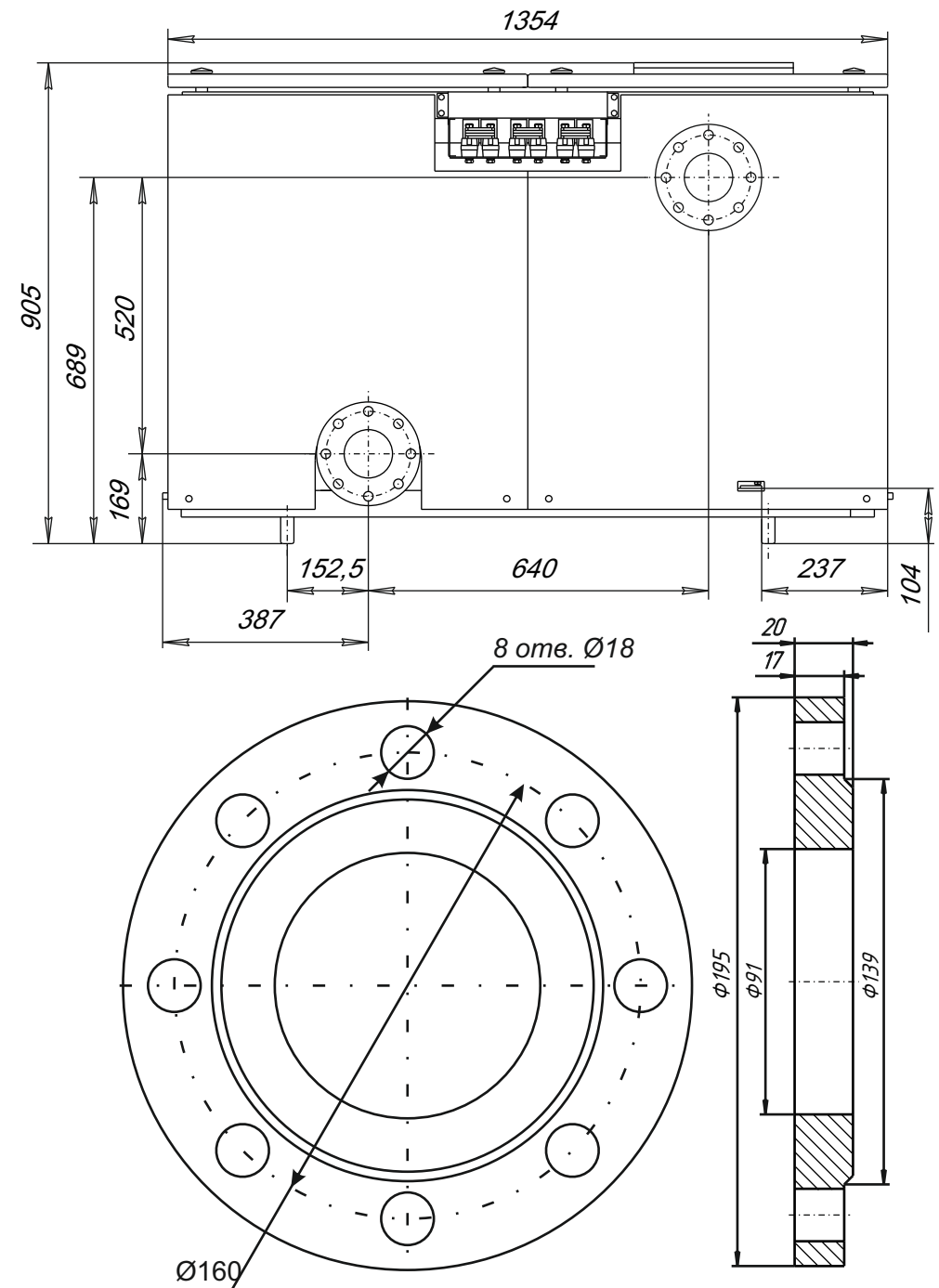
Рис. 4 Вид сзади
