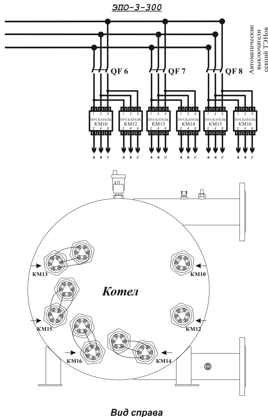
Рис. 9-2 Электрическая схема подключения
