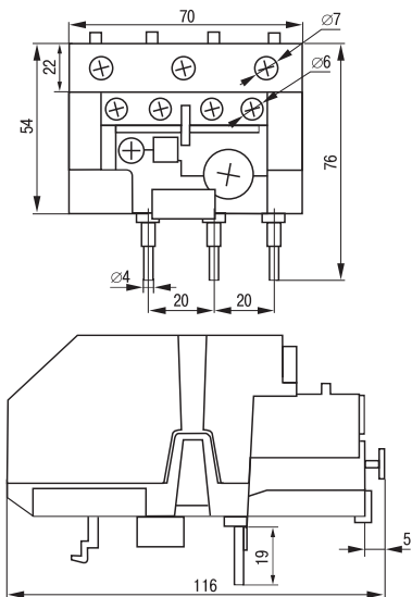
Рисунок 4. Габаритные и установочные размеры реле РТИ-3353...РТИ-3365
