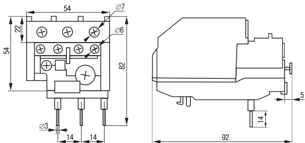
Рисунок 3. Габаритные и установочные размеры реле РТИ-2355
