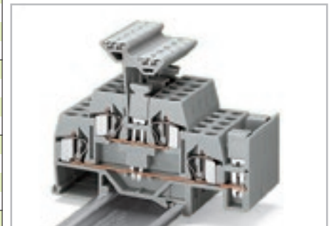
Объединение перемычками двухуровневых клемм
