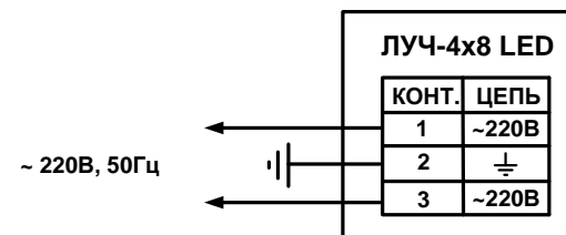
Рис.1. Схема подключения.
