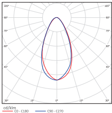
Угол излучения 60°
